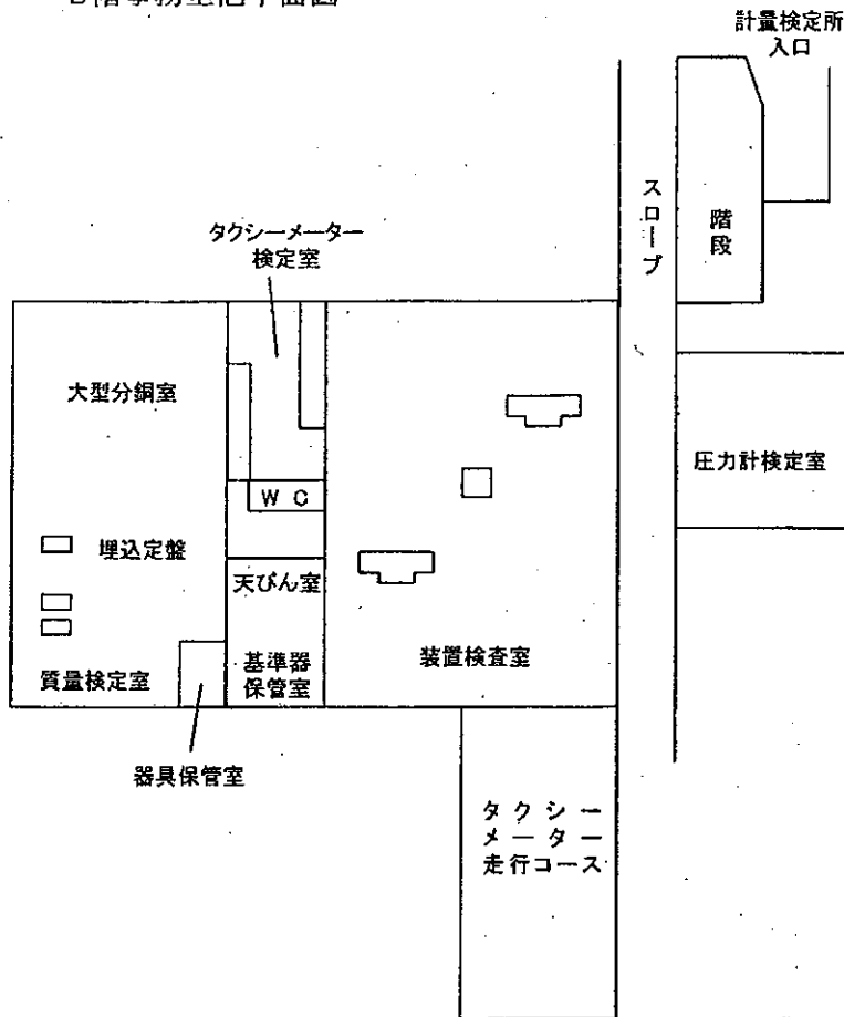
1階検定検査室平面図
