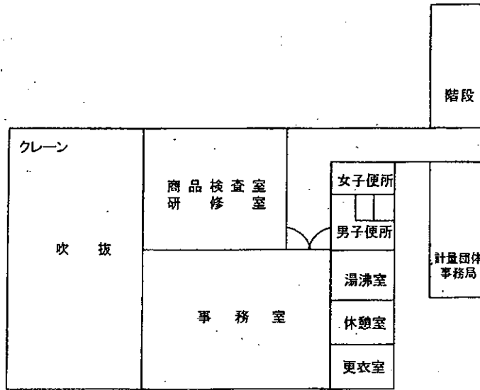
2階事務室他平面図
