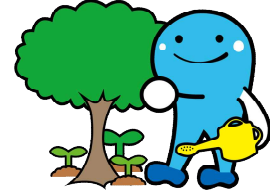
142. グリーン化
