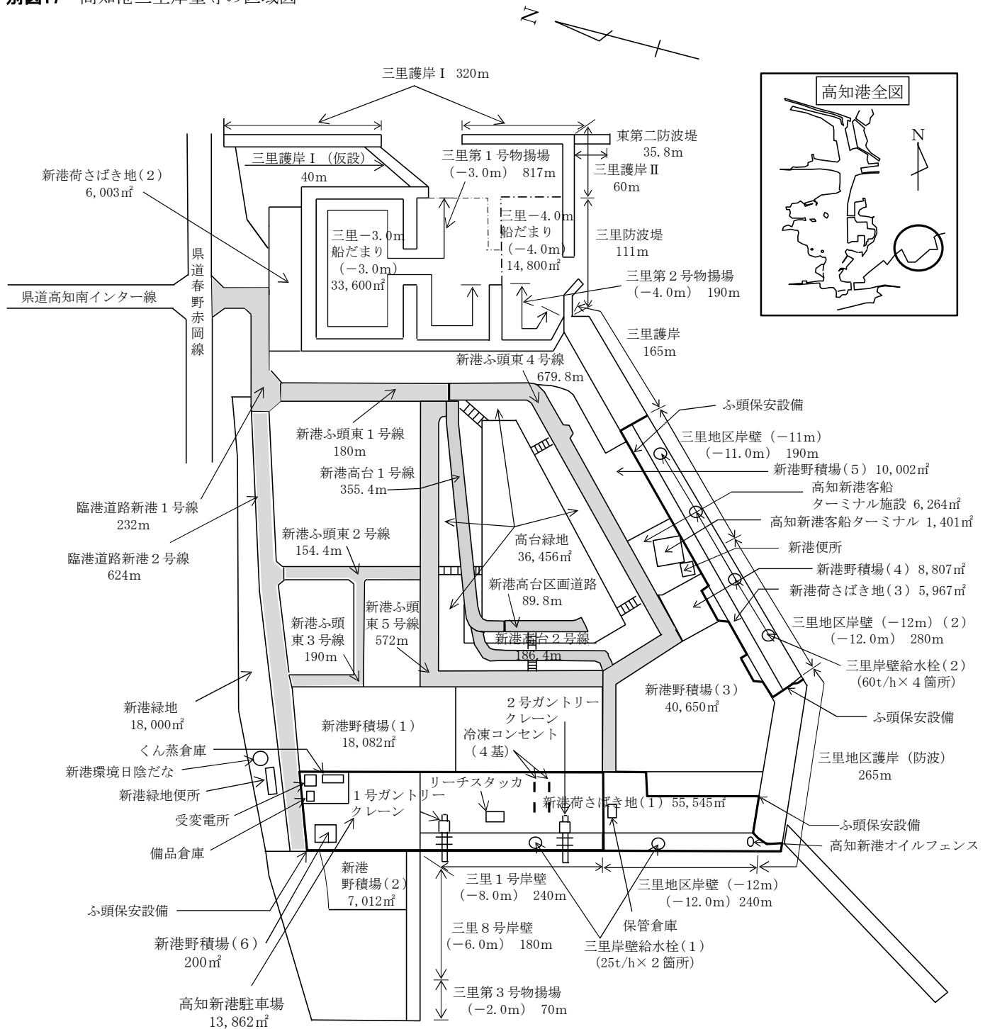
別図17 高知港三里岸壁等の区域図
