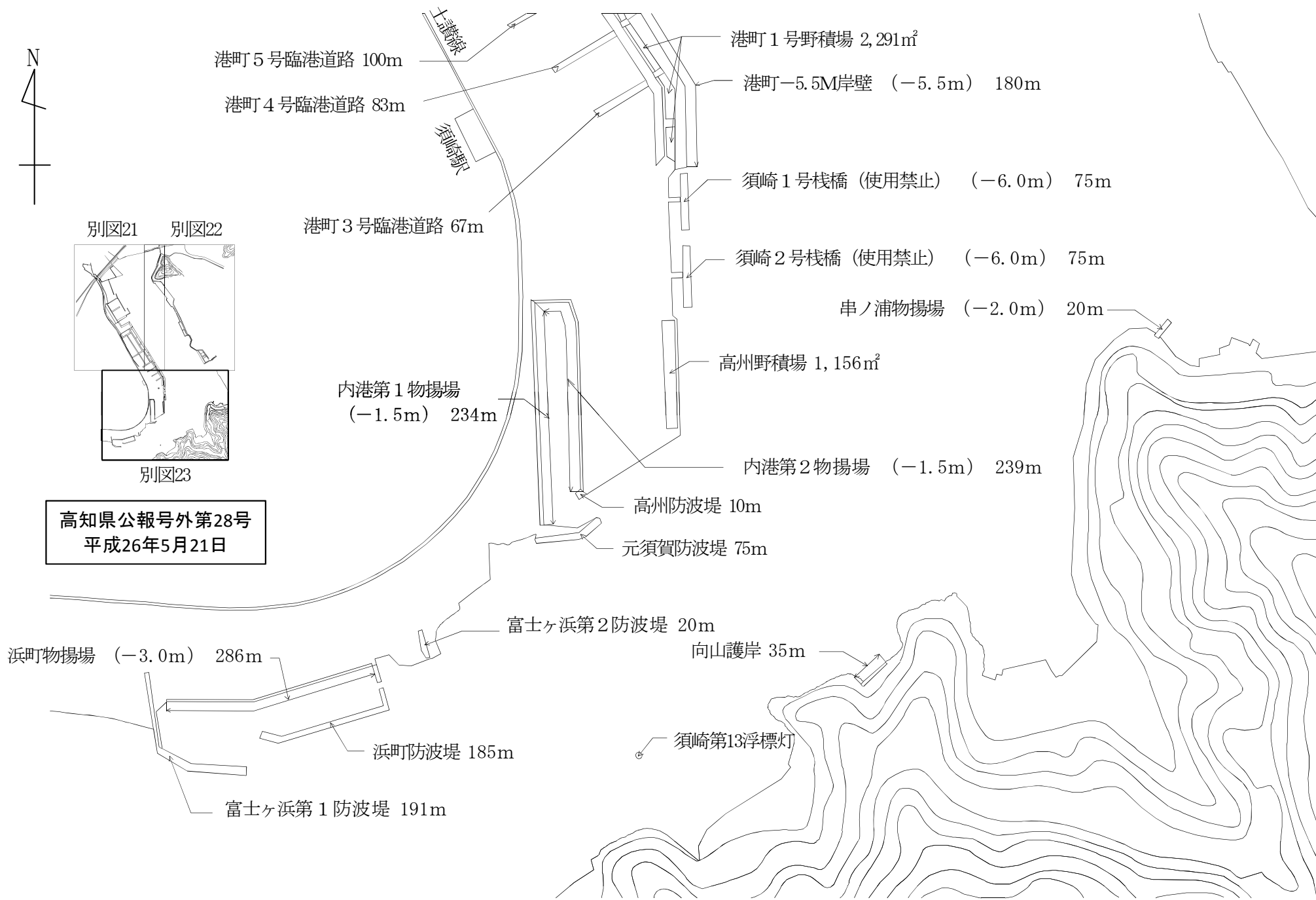
別図23 須崎港浜町物揚場等の区域図
