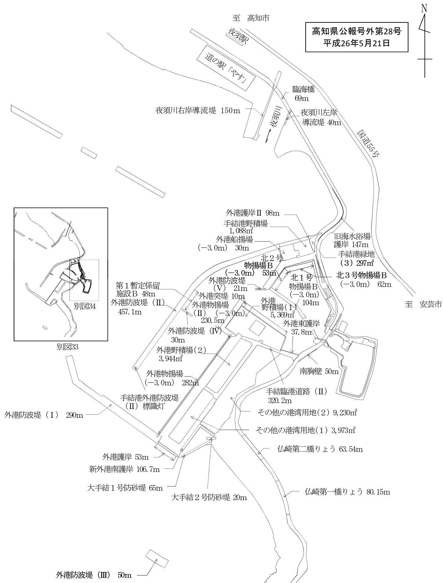
別図33 手結港外港物揚場等の区域図
