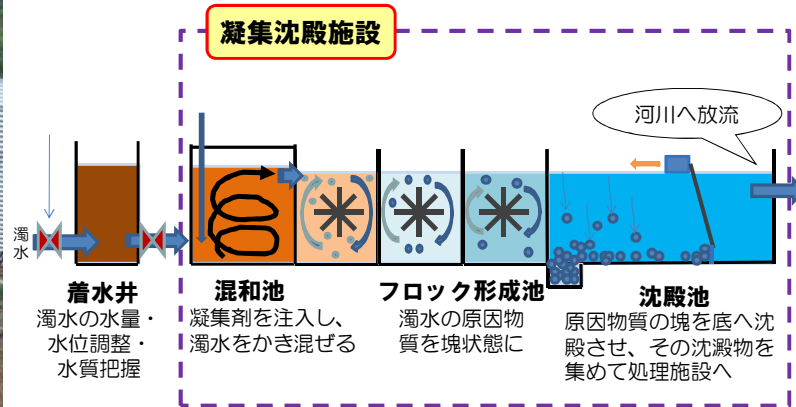
濁水プラントでの処理イメージ
