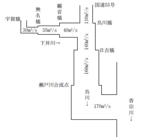
【烏川 流量配分図】
