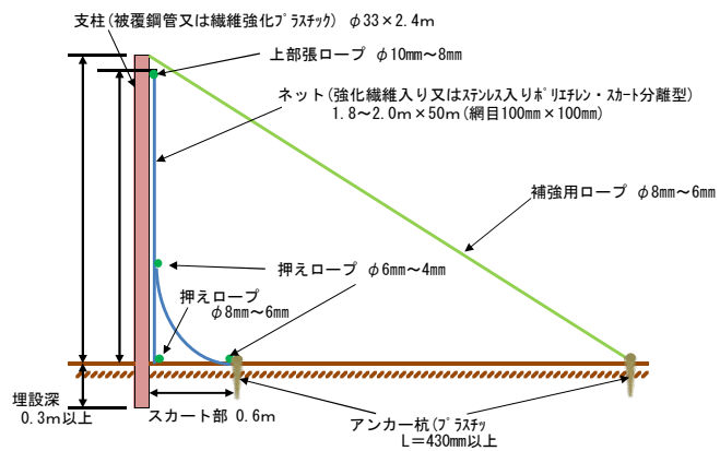
側面図
