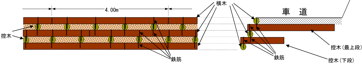
正面図 3段組
