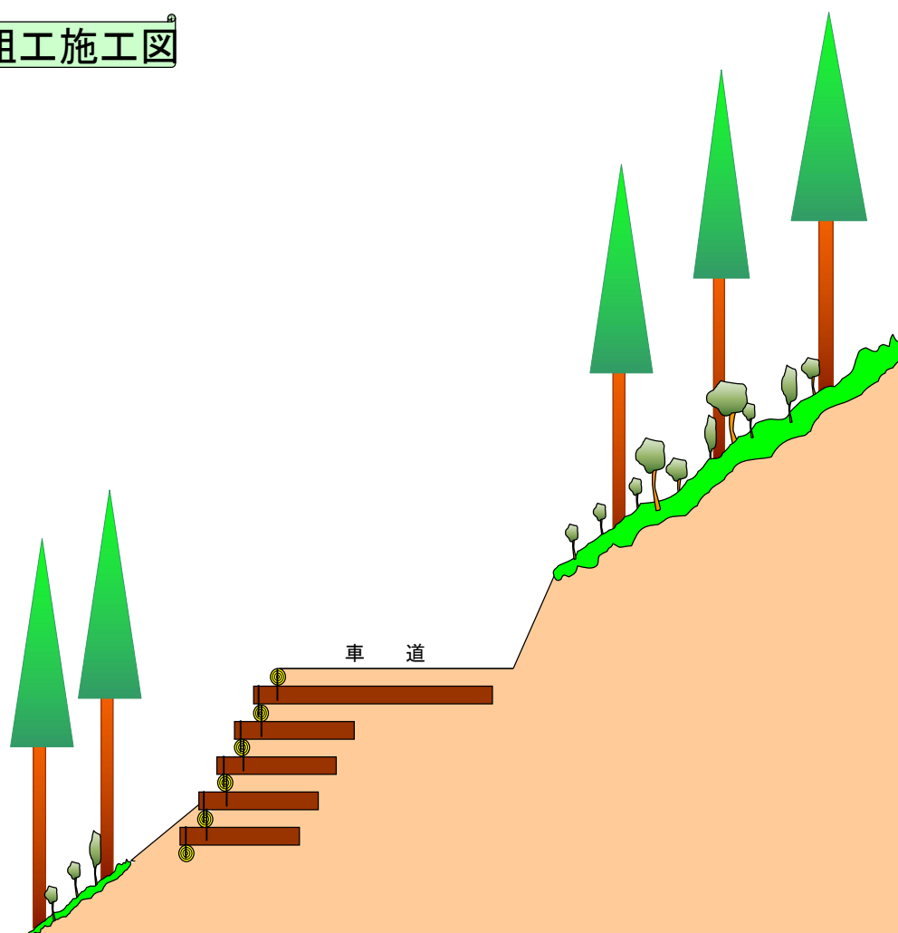
正面図 3段組
