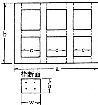
(4本配筋の例)
