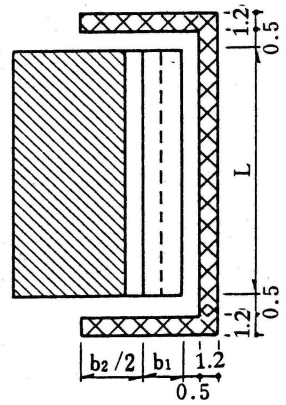
③ 平面図
