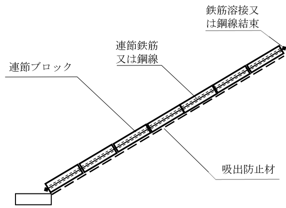
断面図
